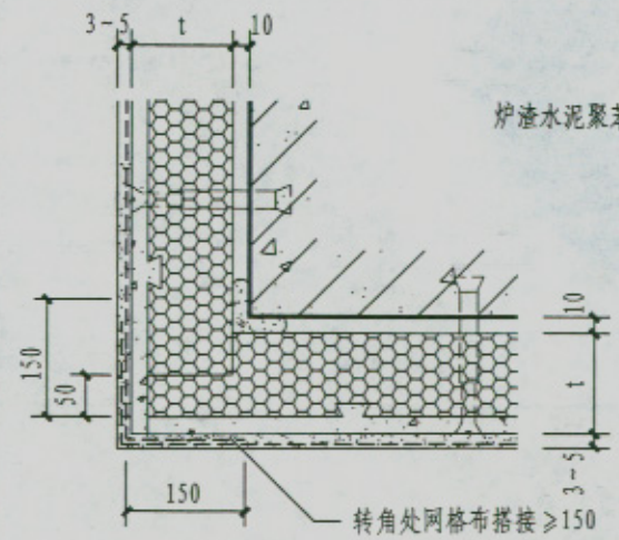
1 做法示意
