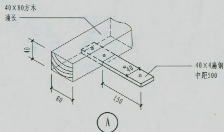
凸(飘)窗节点详图(一)
