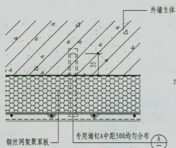
① 与实体墙固定
