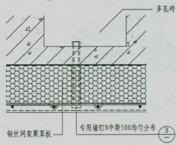
① 与实体墙固定
