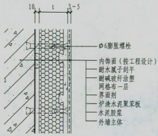
1 做法示意
