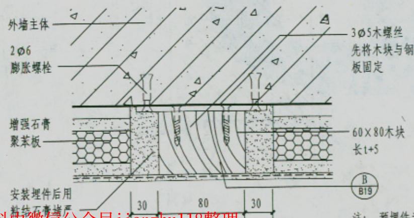
① 埋件做法
