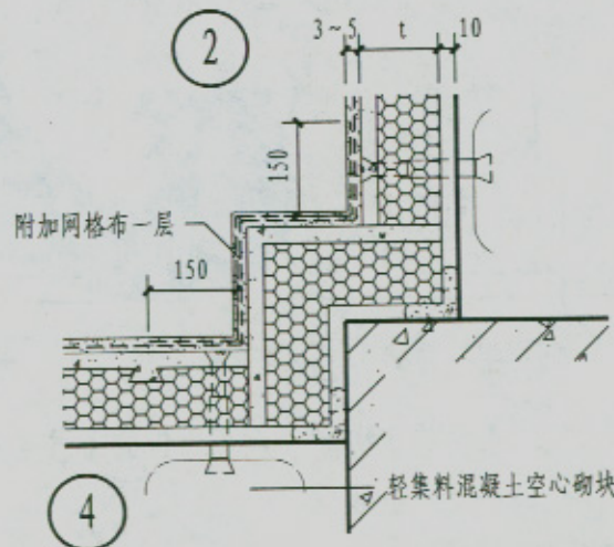
平面节点详图 (三)
