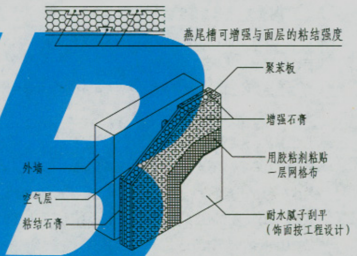
增强石膏聚苯复合板内保温构造示意
