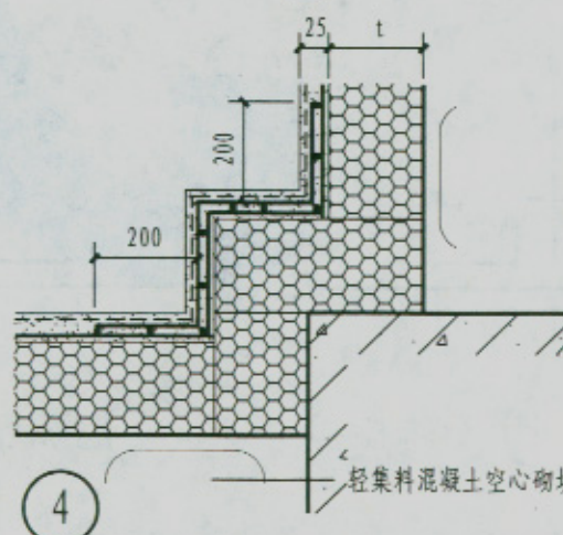
平面节点详图 (三)
