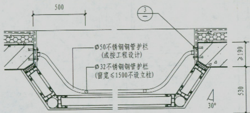
凸窗平面 (以类型C为例)
