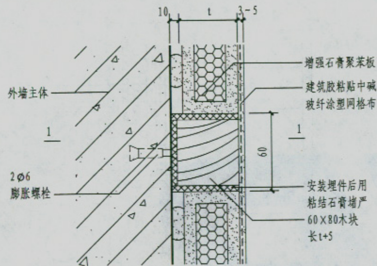
① 埋件做法
