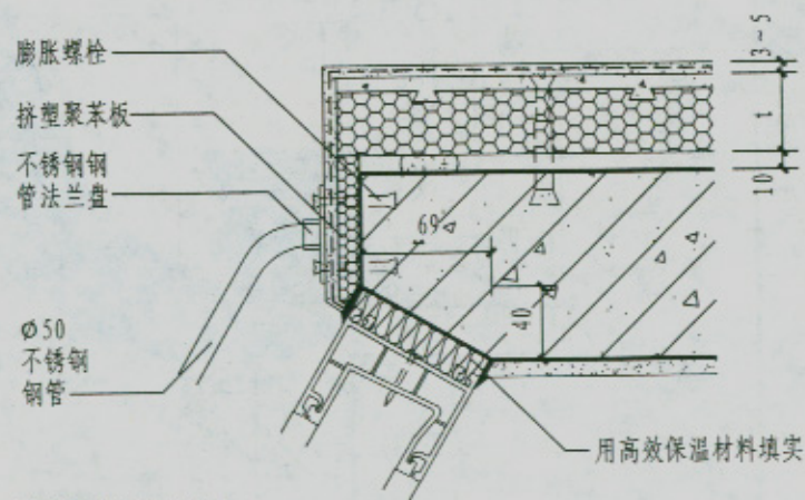
凸窗平面 (以类型C为例)
