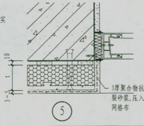
楼层处及窗侧口节点详图
