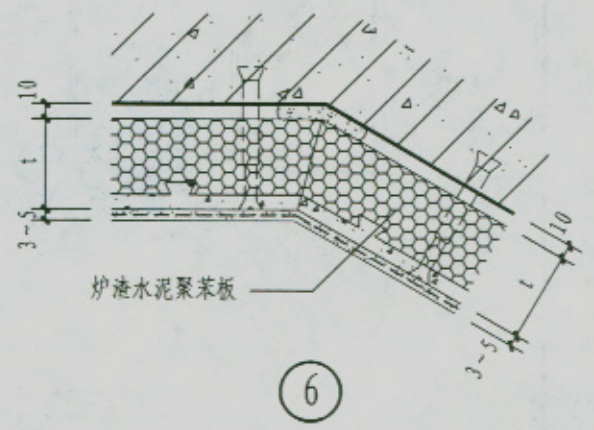
平面节点详图 (一)
