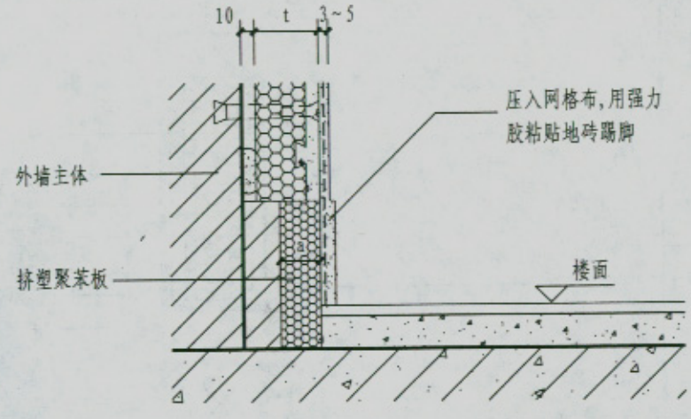
② 地砖踢脚
