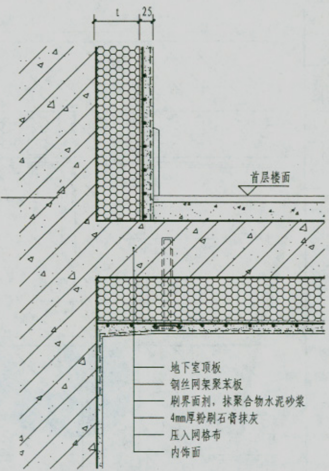
③ 地下室顶板保温 (不采暖地下室)
