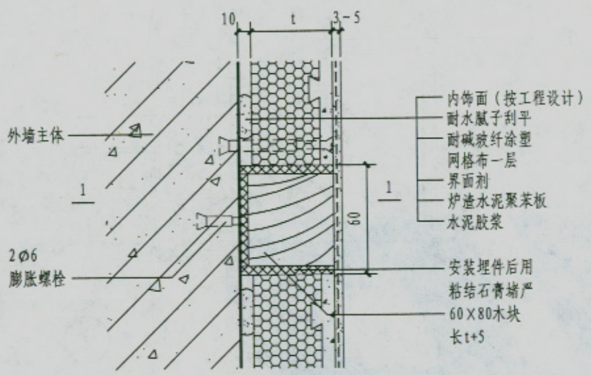
1 埋件做法
