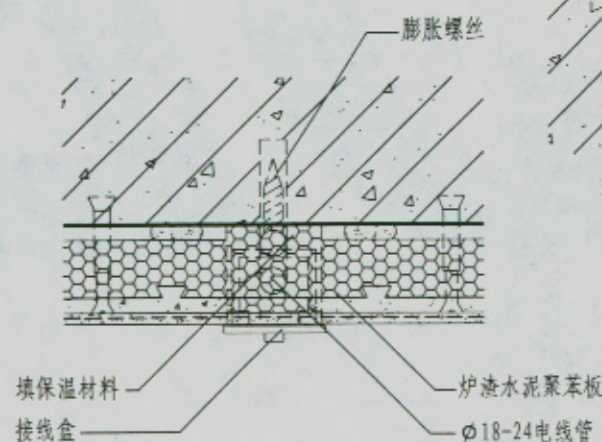
暖气片、开关盒、管卡安装详图
